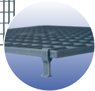
detail: snap-on-leg
